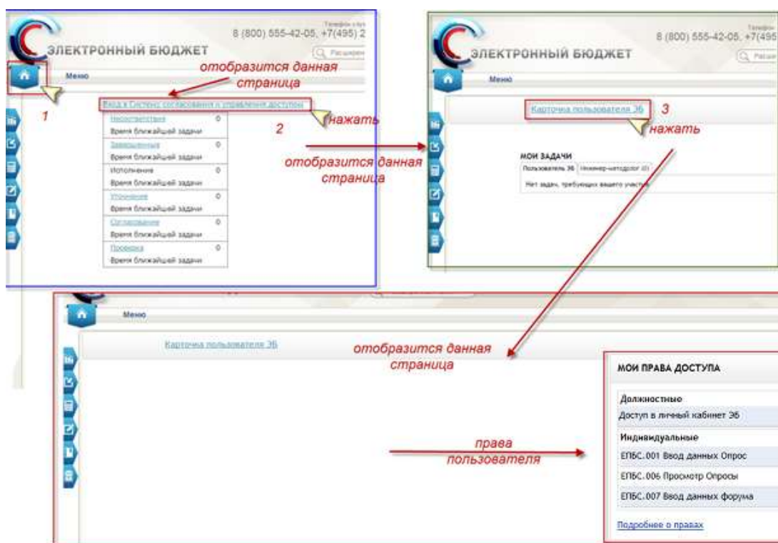
Рисунок 4 – Проверка полномочий
